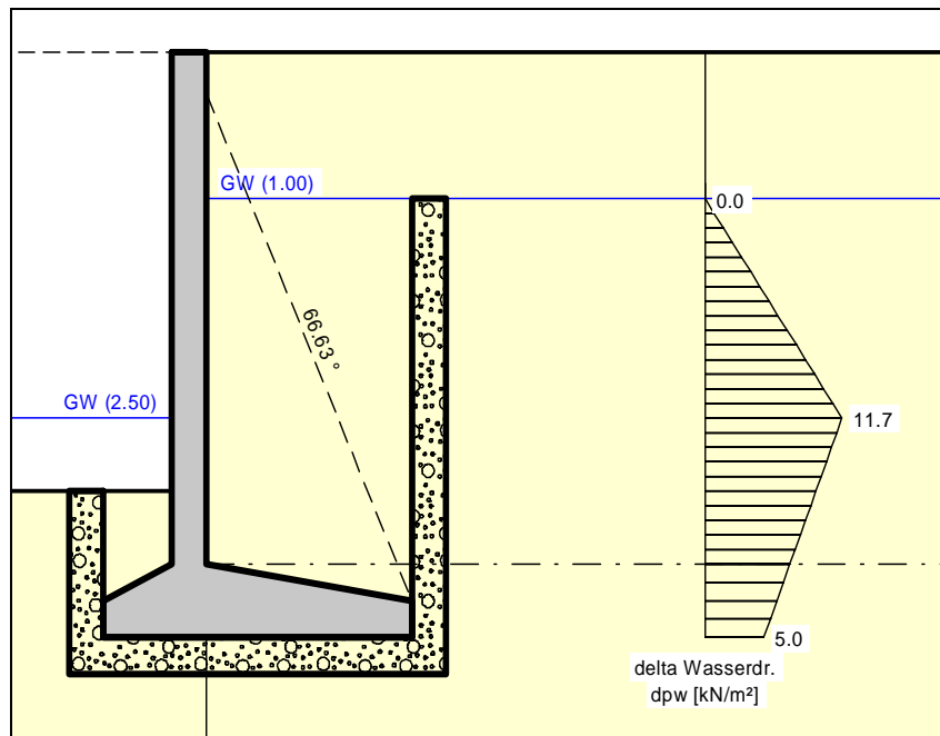
Abbildung 9 Resultierende Wasserdruckbelastung mit Stromröhren
