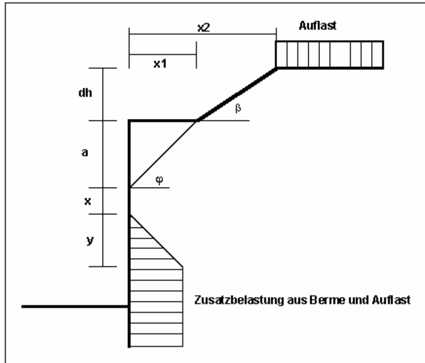
Abbildung 11 Berme auf der Aktivseite
