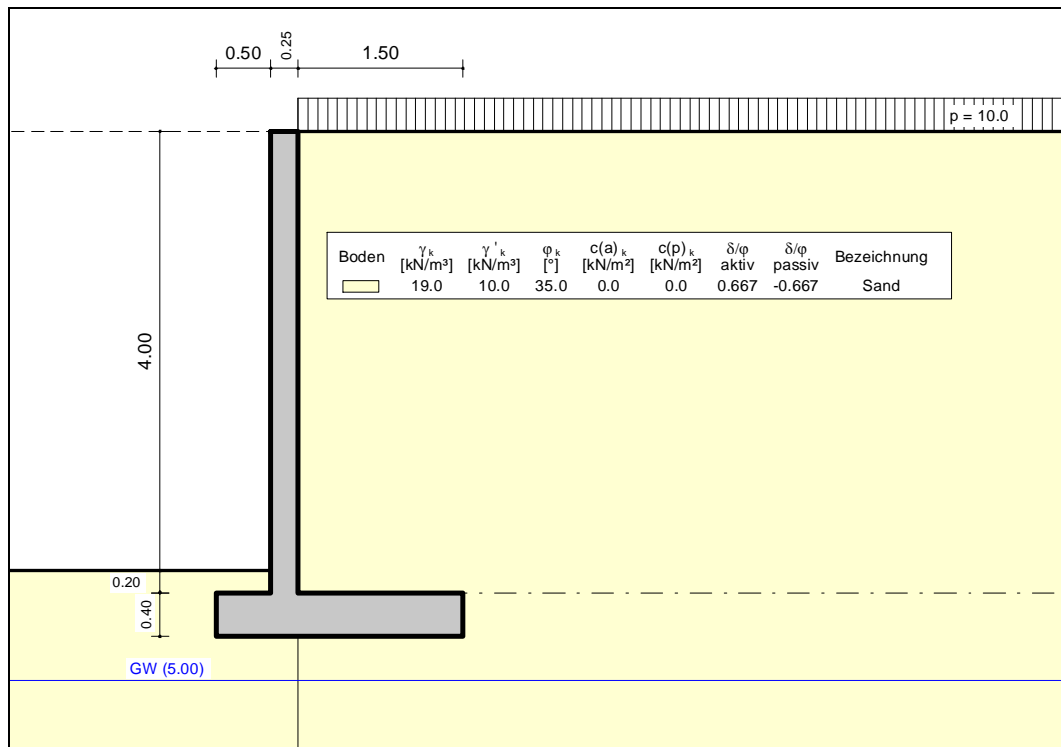
Abbildung 1 Beispielsystem für Kurzeinführung
