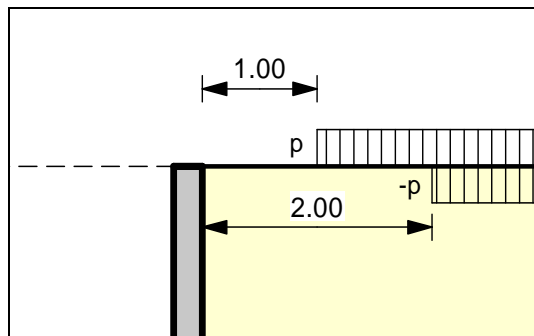
Abbildung 15 Zwei einseitig begrenzte Lasten
