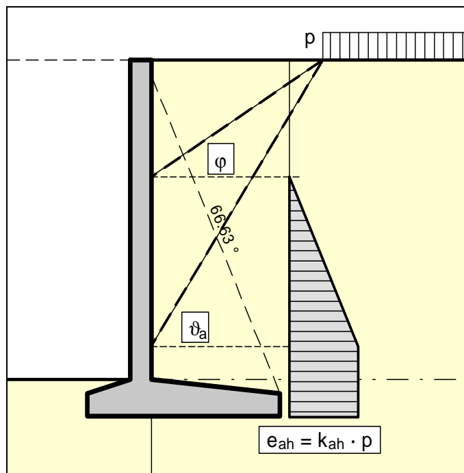
Abbildung 14 Einseitig begrenzte Last (Aktivseite)
