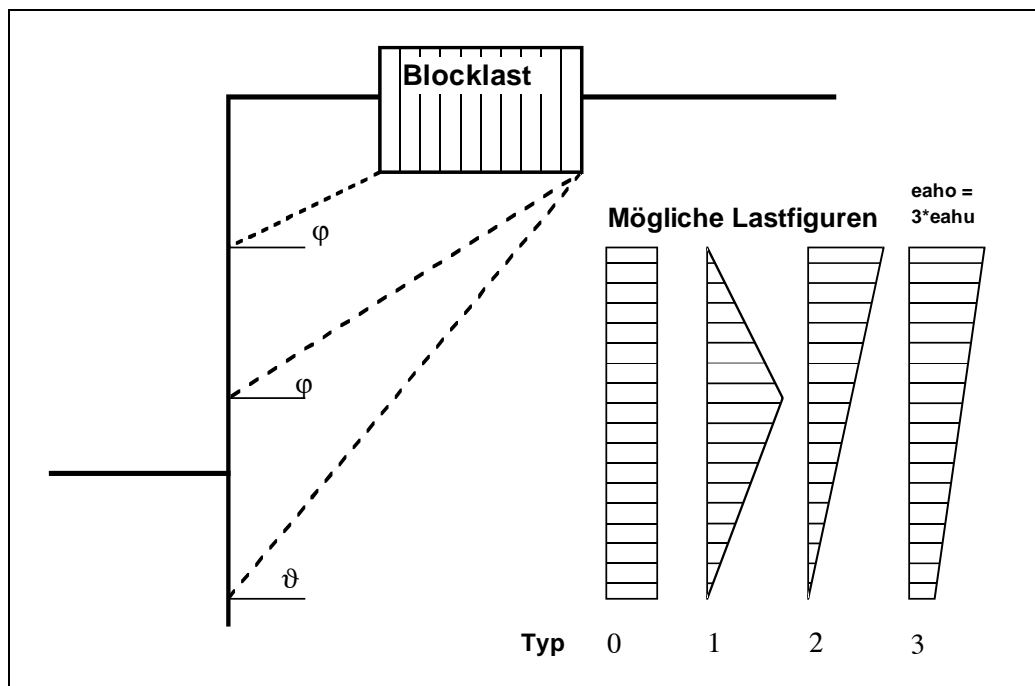
Abbildung 12 Blocklast
