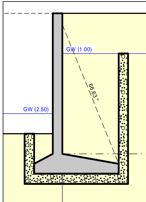
Abbildung 8 Wasserdruckansatz mit Stromröhre
