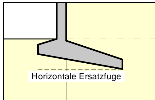
Abbildung 19 Horizontale Ersatzfuge
