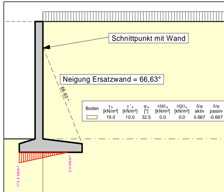
Abbildung 4 Neigung Ersatzwand
