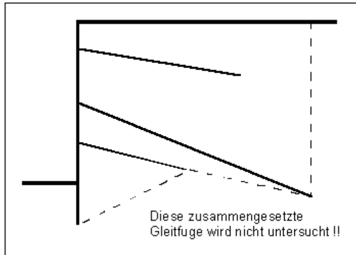
Abbildung 21 Zusammengesetzte "Tiefe Gleitfuge", die nicht untersucht wird
