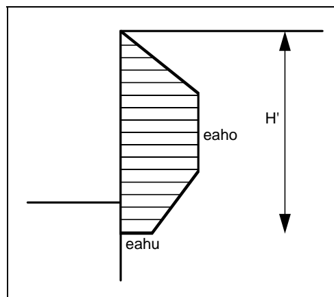
Abbildung 24 Erddruckumlagerung in ein Viereck
