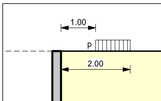
Abbildung 16 Zweiseitig begrenzte Last
