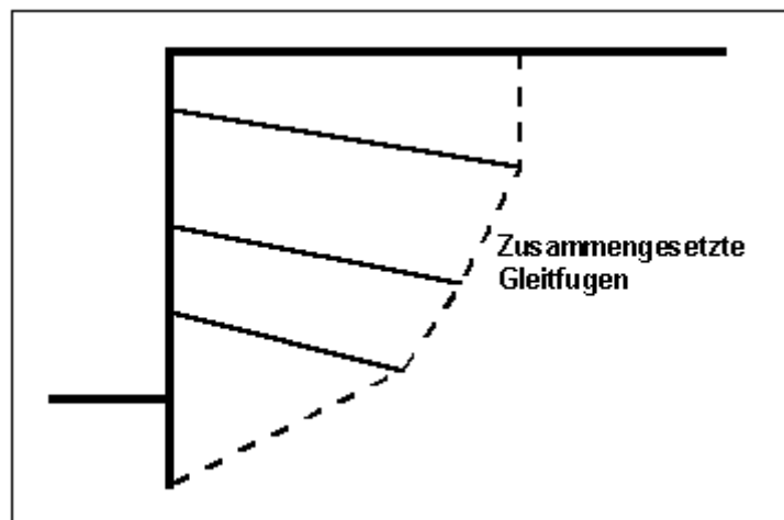
Abbildung 20 Zusammengesetzte "Tiefe Gleitfugen"
