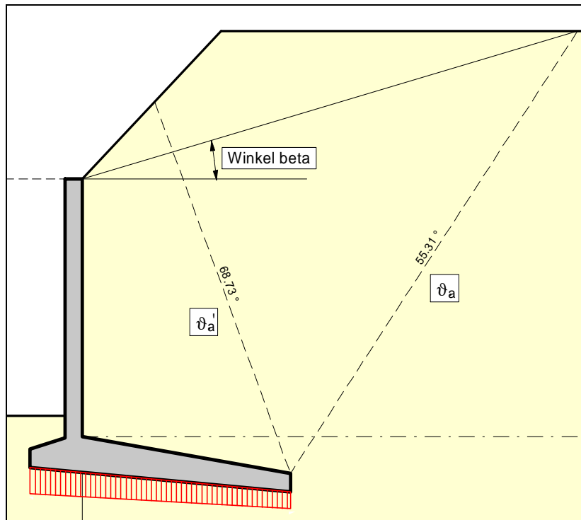
Abbildung 5 Ermittlung des Winkels \beta
