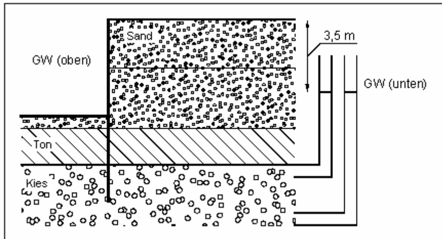
Abbildung 10 Potentialdefinition
