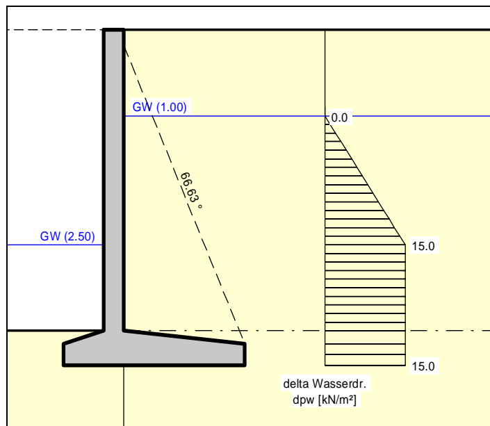
Abbildung 7 Resultierende Wasserdruckbelastung
