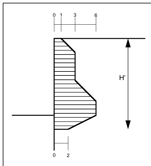
Abbildung 25 Beliebige Erddruckumlagerung
