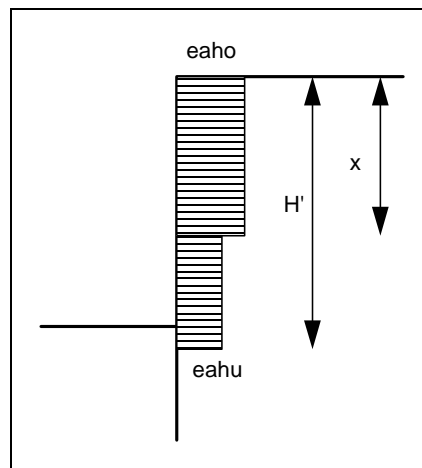
Abbildung 22 Erddruckumlagerung in 2 Rechtecke
