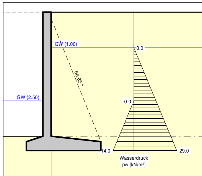
Abbildung 6 Herkömmlicher Wasserdruckansatz
