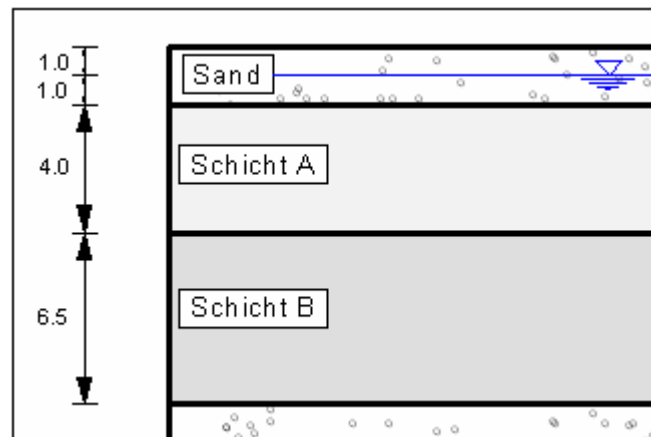
Abbildung 7 Ausschnitt Beispielsystem
