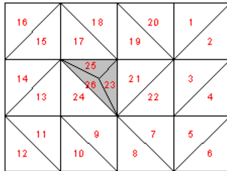
Abbildung 3 Verdichtung FE-Netz mit Verfahren 1
