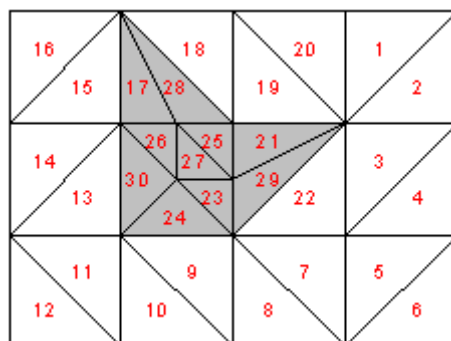
Abbildung 5 Verdichtung FE-Netz mit Verfahren 3
